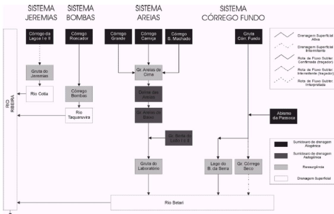
Figura 1 – Rotas de Fluxo identificadas na Faixa Lajeado/Bombas utilizando traçador fluorescente Rodamina-WT
