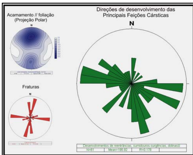
Figura 6.8 - Em verde, diagrama de rosetas, unidirecional, indicando as direções de desenvolvimento das principais feições cársticas. Direções preferenciais para WNW e para SSE, paralelas a subparalelas as direções dos trends estruturais: fraturas e acamamento/foliação.
