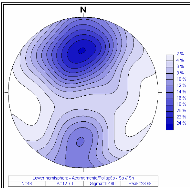
Figura 6.2 - Estereograma de concentração das projeções polares dos acamamentos (So), bem como foliações paralelas a ele.
