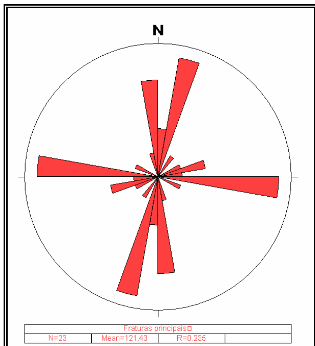
Figura 6.5 - Diagrama de rosetas, bidirecional, das direções de fraturas medidas no campo. Observam-se as direções WNW-ESSE e NNE-SSW como sendo as principais.
