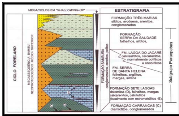
Figura 5.1 - Coluna Estratigráfica do Grupo Bambuí, modificado de Martins-Neto e Alkmim, 2001. Nesta figura acrescenta-se a subdivisão apresentada in Dardene & Schobbenhaus (2000).
