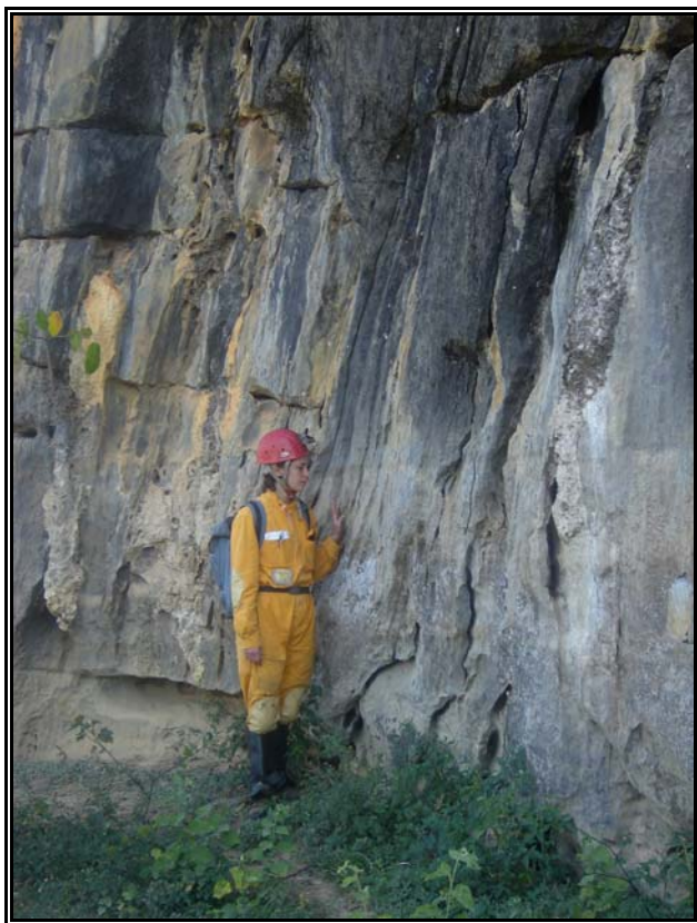
Figura 6.4 - Foliação subverticalizada de maciço calcário - Ponto MS - 78.
