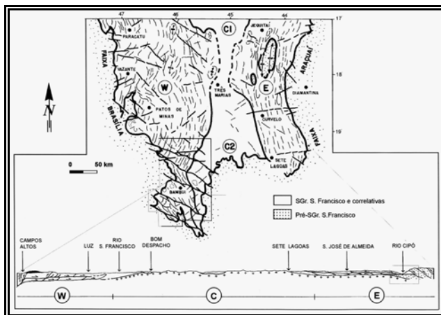
Figura 5.2: Mapa dos domínios estruturais da parte sul da Bacia do São Francisco (segundo Martins-Neto e Alkmim 2001).
