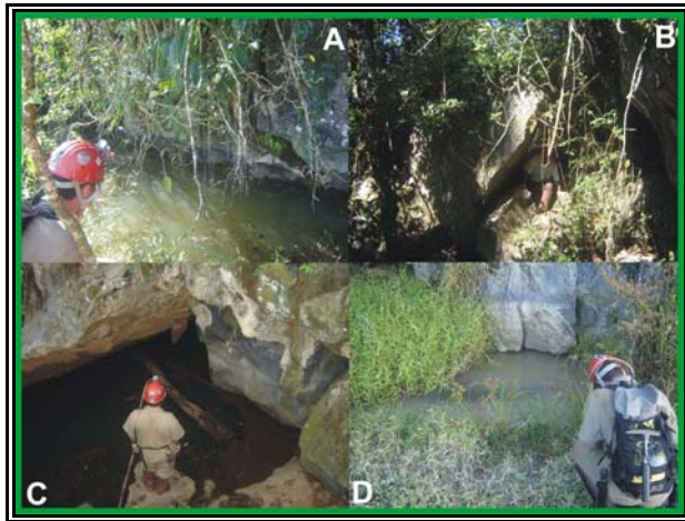
Figura 6.7 - Quatro cenários típicos da paisagem cárstica dos Maciço Sul. A) ponto MS - 80, sumidouro perene; B) ponto MS - 101 - aspecto ruiniforme, matacões com abrigo sob eles; C) ponto MS - 147 - sumidouro perene, detalhe de tronco de árvore flutuando em lago adjacente ao maciço e D) ponto MS 161 - surgência perene.
